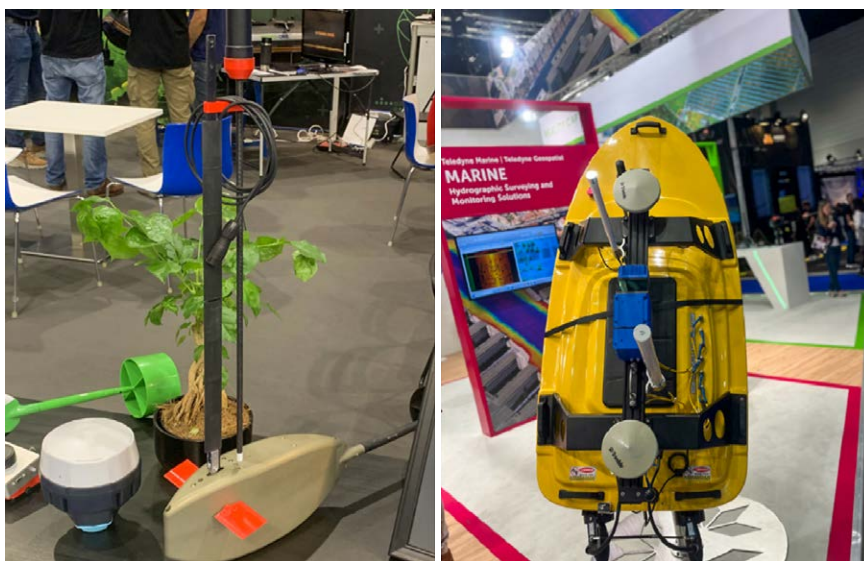
Auf der linken Seite ist eine Drohnenlösung für die bathymetrische Vermessung zu sehen, auf der rechten Seite ein Hydrologie-Einsatzfahrzeug.
