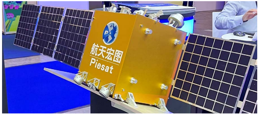
Ein Modell des inSAR-Satelliten PIESAT 1A-01, welcher zur inSAR-Konstellation gehört, die aus aktiven und passiven X-Band-SAR-Satelliten besteht. Die Konstellation wird Daten mit einer Auflösung von bis zu 0,5 m für die Untersuchung und frühzeitige Erkennung bedeutender geologischer Gefahren wie Bodensenkungen, Einstürze und Erdbeben liefern.
