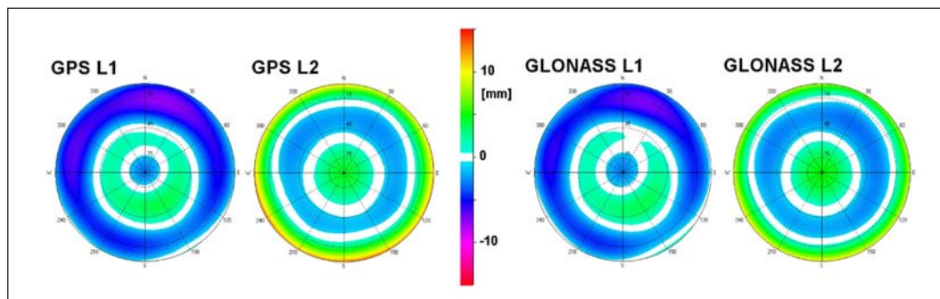
Abb. 1: Signalfrequenz- abhängige Antennen- kalibrierergebnisse einer GPS/GLONASS- Antenne für alle Signaleinfallswinkel
